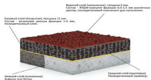
Покриття CONIPUR SP в розрізі
